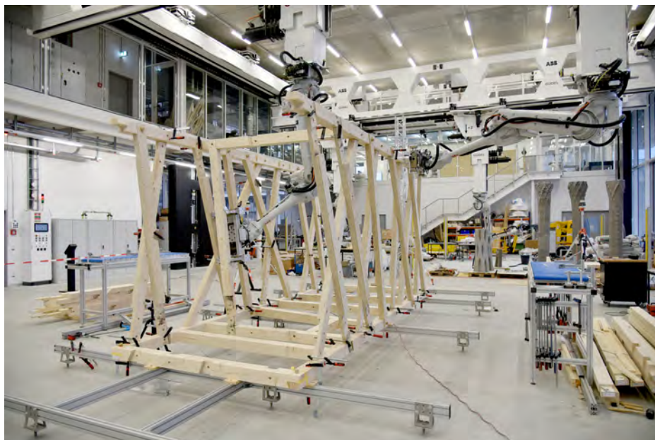
木造骨組みモジュールは、ETHチューリヒのロボティック・ファブリケーション・ラボでプレハブ工法を用いて建設された。 © Gramazio Kohler Research, ETH Zurich
